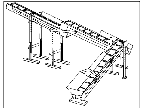
4 Förderbänder mit Glatt- bzw. Stollengurt - kombinierbar, je nach Kundenanforderung
