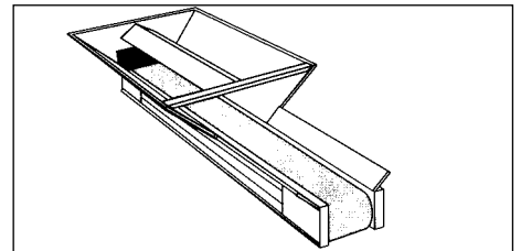
4 Fallbrecher im Aufgabetrichter für geringste Gurtbelastung und bestmögliche Verteilung
