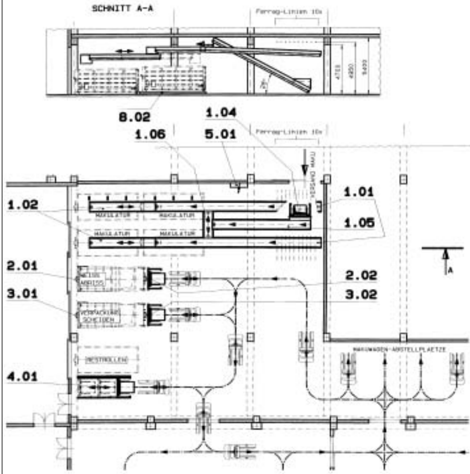
1 Zeichnungsdarstellung einer kompletten Entsorgungsstation in einem Druckzentrum
